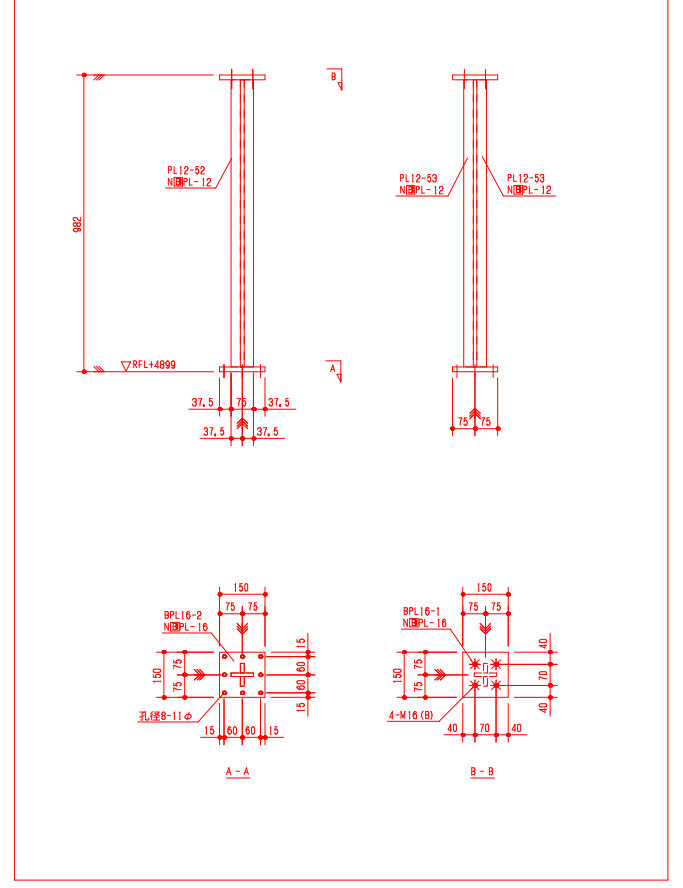
スピーカー受下地製作要領図
