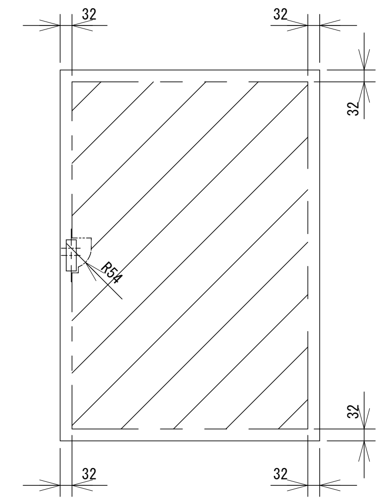
扉 機器取付有効図
